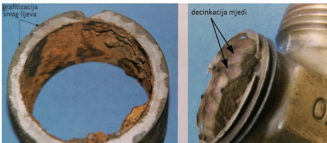
Slika 10. Selektivna korozija [1].
