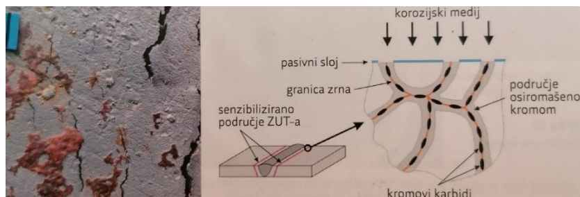
Slika 9 Interkristalna korozija [1].
