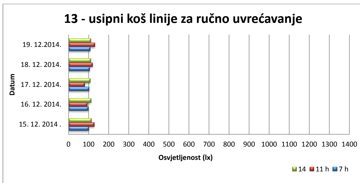
Sl.4.4.2. Grafički prikaz vrijednosti parametara osvjetljenosti za radno mjesto br. 13
