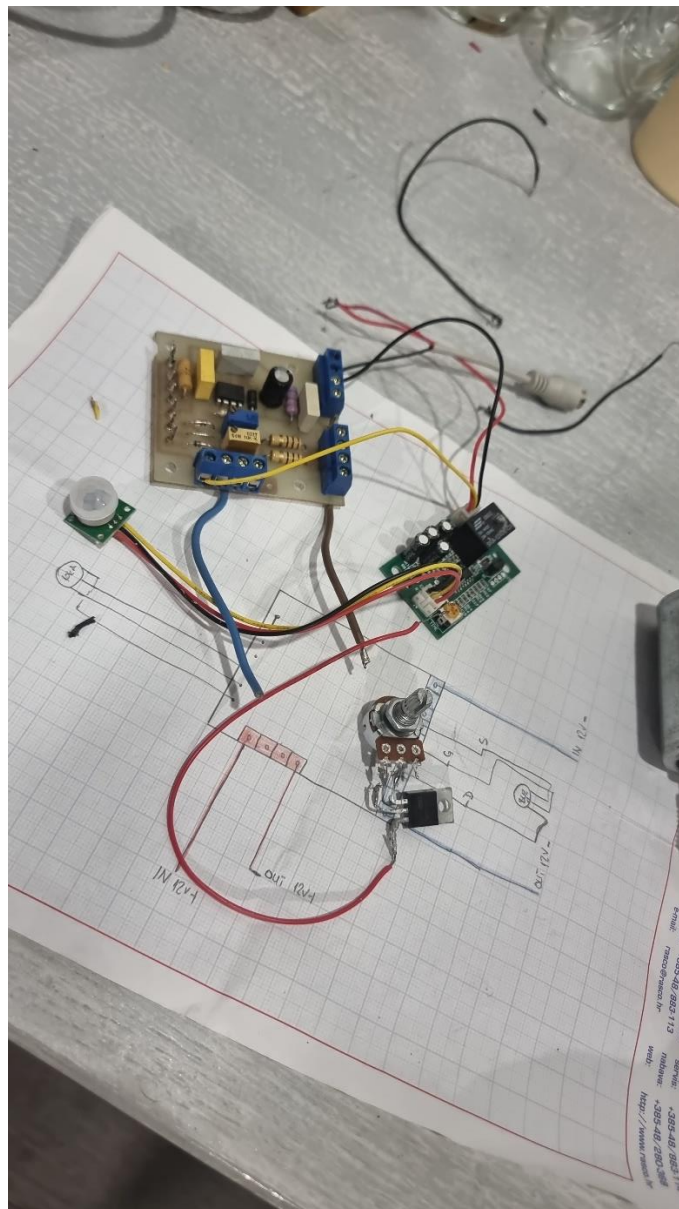
Slika 34. Testiranje sklopa.
