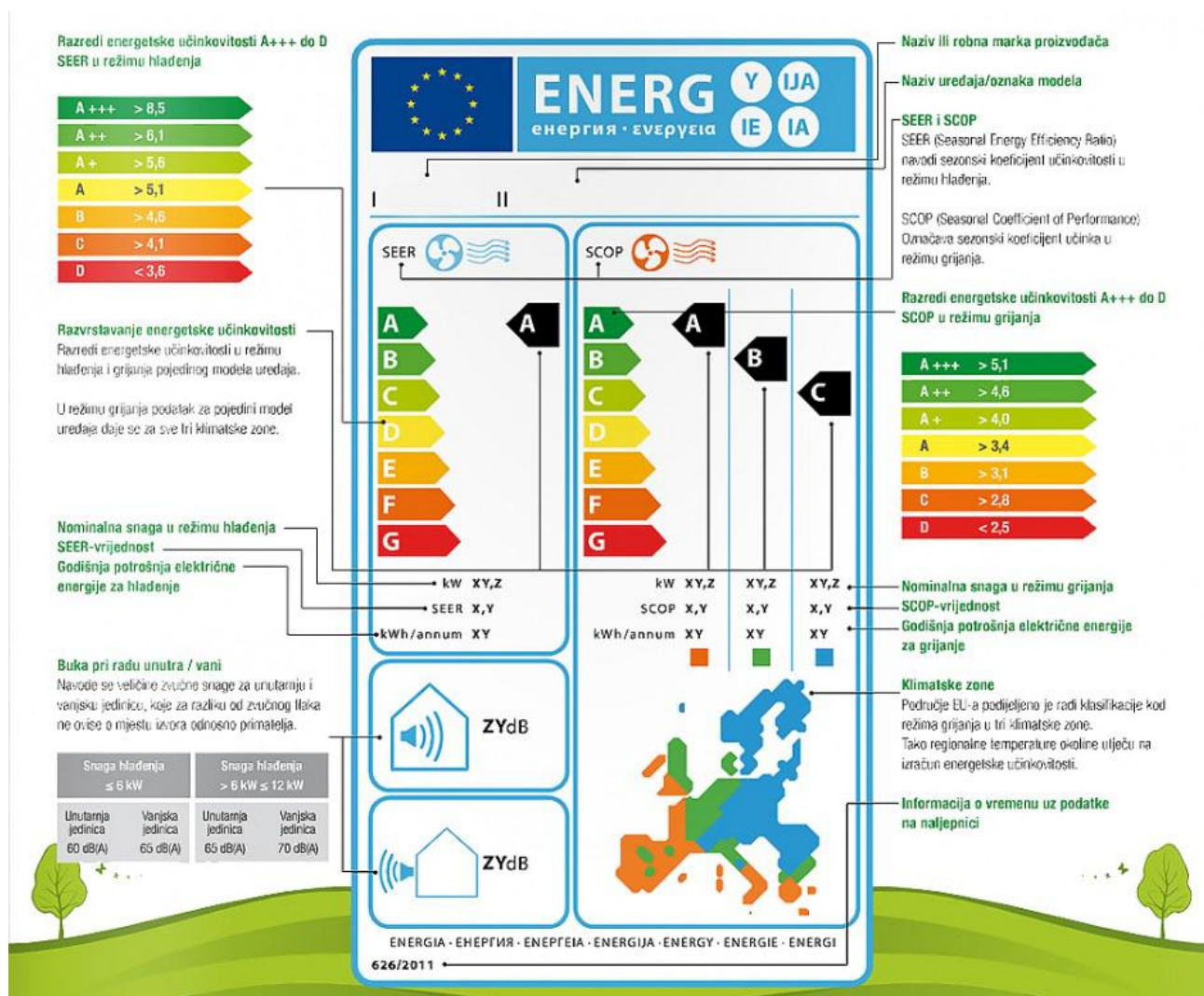
Slika 4.8. Prikaz pojašnjenja podataka na energetske naljepnici [14]
