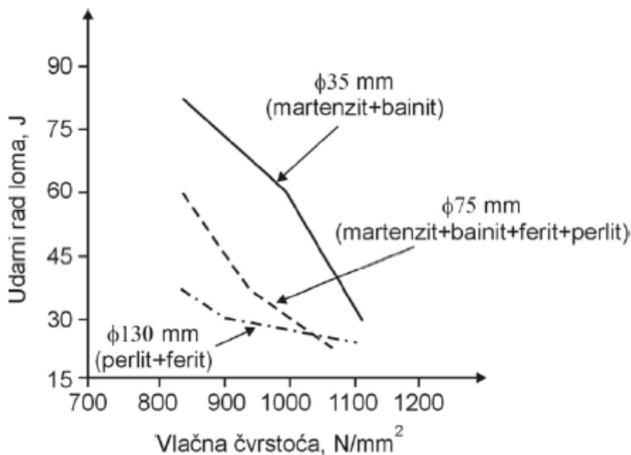
Slika 3.1.5. Utjecaj mikrostrukture nakon gašenja i promjera čelika na vlačnu čvrstoću i udarnu radnju loma ( Č.4830 ) [4]
