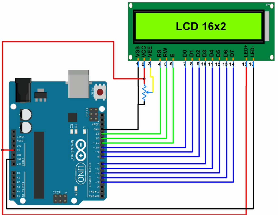
Slika 37. Shema spajanja LCD zaslona i Arduino mikrokontrolera [15]
