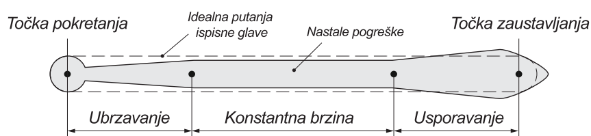
Slika 78. Pogreške u dimenzijama na putanji ispisne glave [79]
