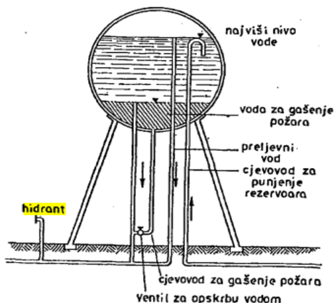
Slika 19. Nadzemni rezervoar – kugla[13]
