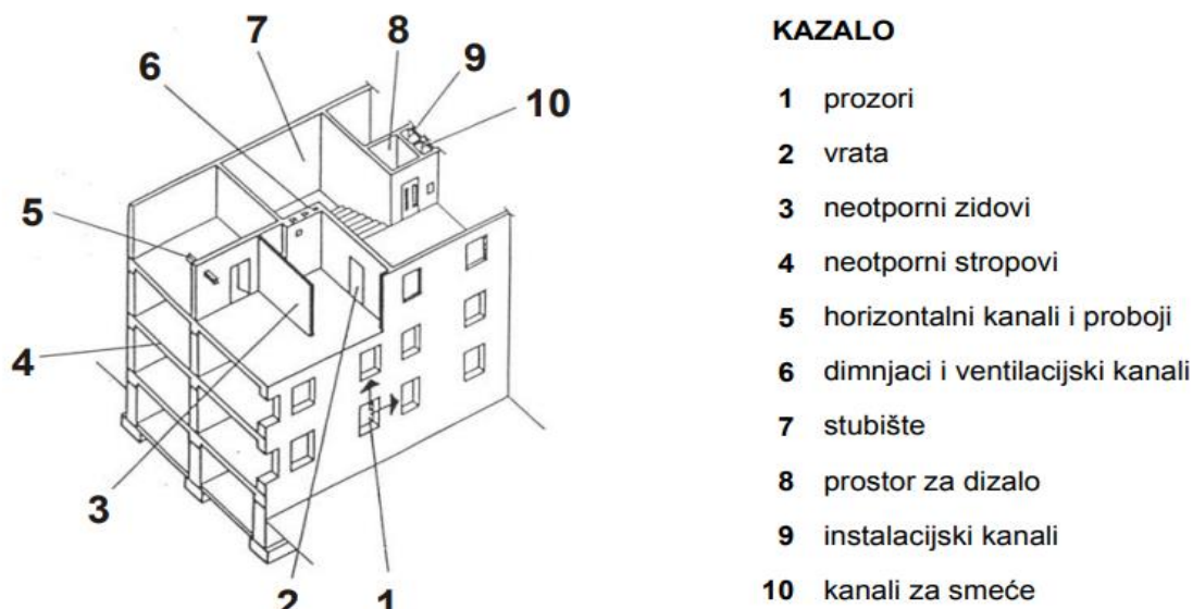
Slika 5. Prikaz putova širenja požara u objektu[6]
