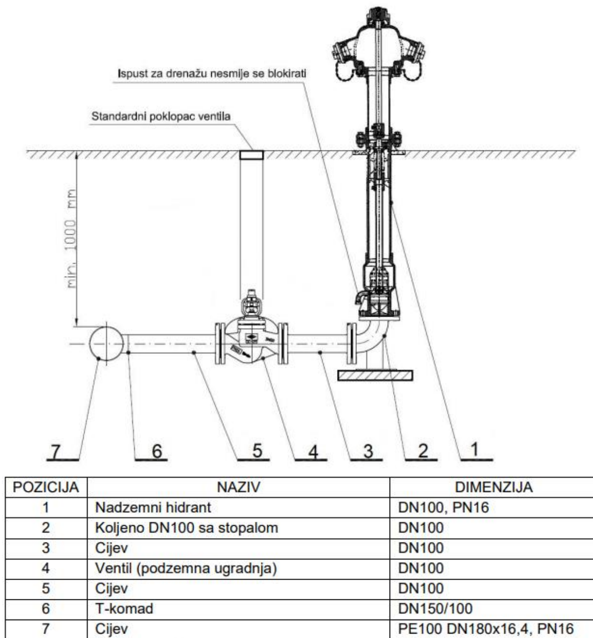
Slika 35. Nadzemni i podzemni hidrant vanjske hidrantske mreže u proizvodnom pogonu poliestera tvrtke „AQUAESTIL PLUS“ [27]
