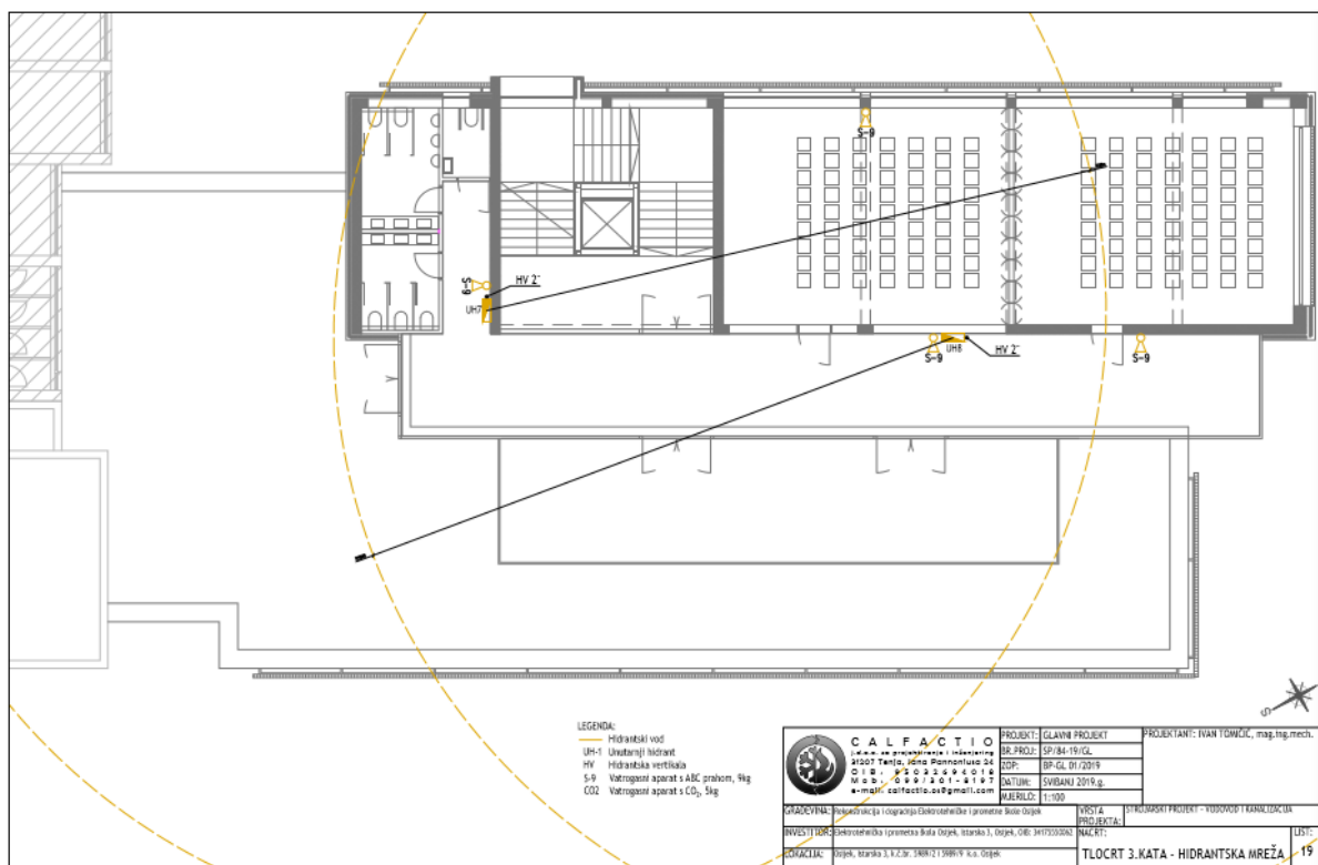
Slika 31. Tlocrt 3. kata zgrade Elektroničke i prometne škole u Osijeku sa rasporedom hidrantskih ormarića[26]
