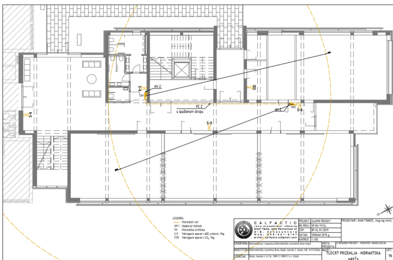
Slika 28. Tlocrt prizemlja zgrade Elektroničke i prometne škole u Osijeku sa rasporedom hidrantskih ormarića[26]
