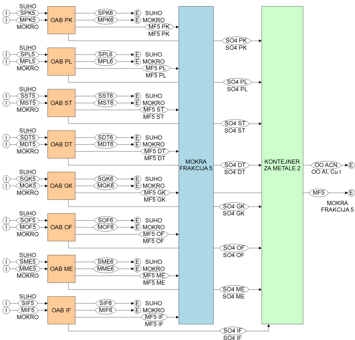
Slika 82. Blok shema podsustava odvajaa aluminija i bakra.
