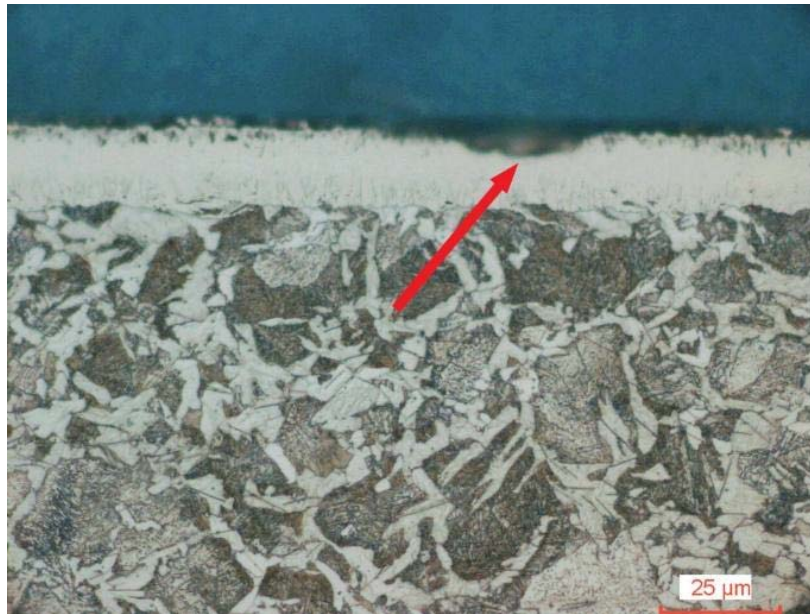
Slika 10. Deformacija nitridnog sloja vidi se na mjestu gdje se gubi fokus fotografije [22]
