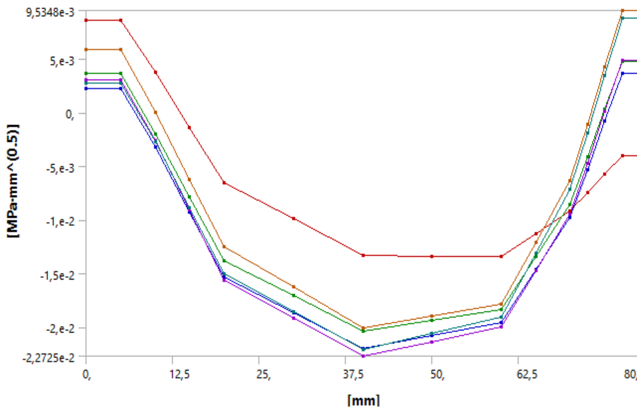
Slika 27 Koeficijent K_I
