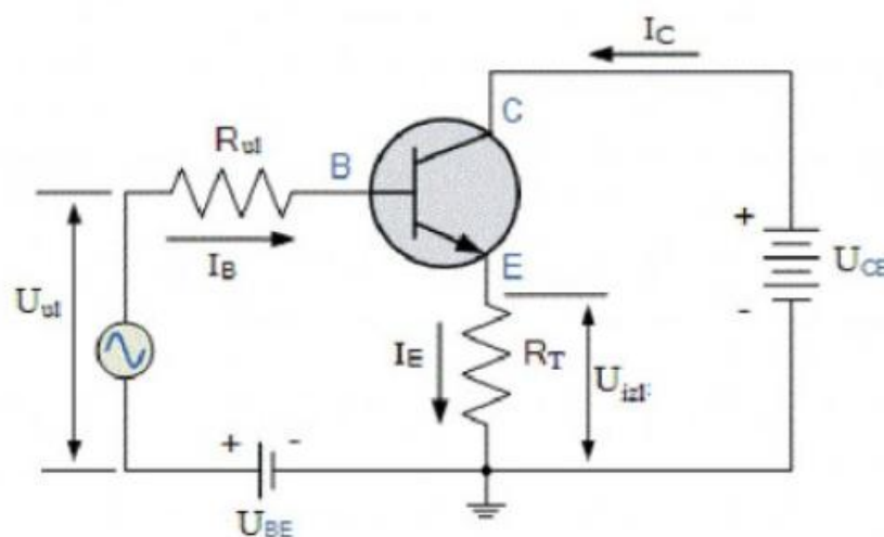
Slika 5. Predodžba tranzistorskog spoja s zajedničkim kolektorom
