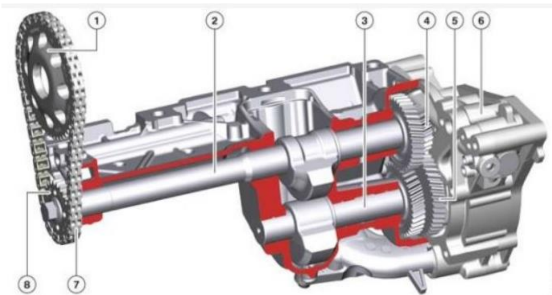
Slika 58. Presjek motora s rotirajućim osovinama za uravnoteženje vibracija [6]
