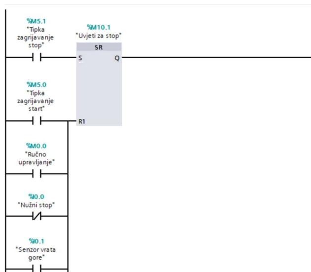
Slika 25. Uvjeti za gašenje grijača (izvorno autor)
