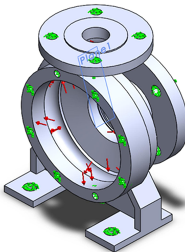
Slika 17 Prikaz modela sa postavljenim opterećenjem
