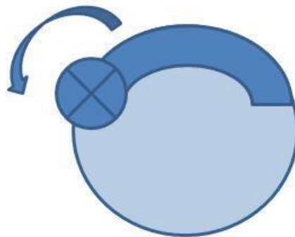
Slika 8. Vanjsko kružno pravocrtno glodanje [7]
