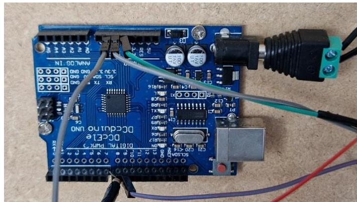
Slika 19. Arduino UNO
