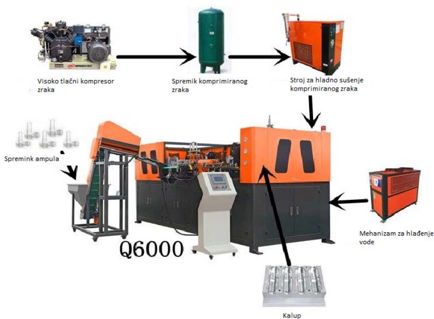
Slika 7: Stroj za izradu boca [9]
