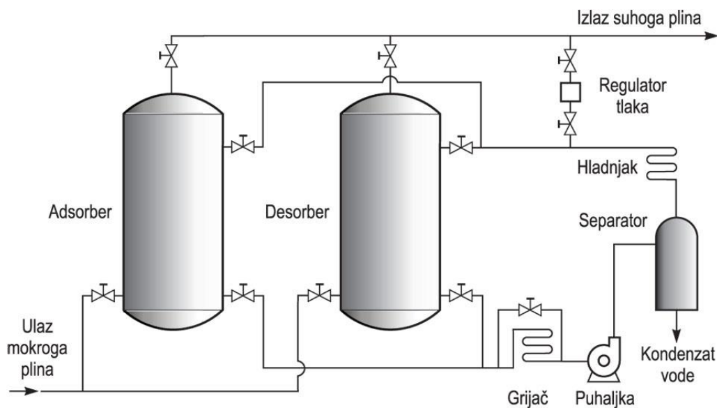
Slika 13. Metoda adsorpcije [18]
