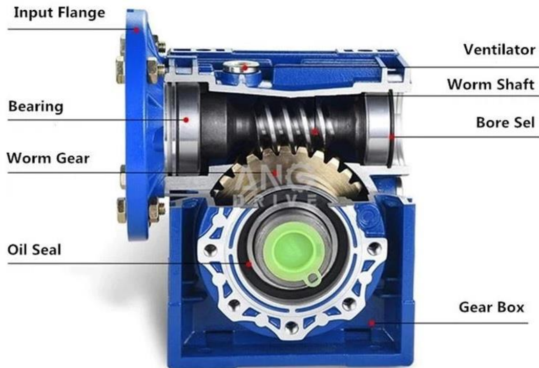
Slika 16. Pužni reduktor [23]
