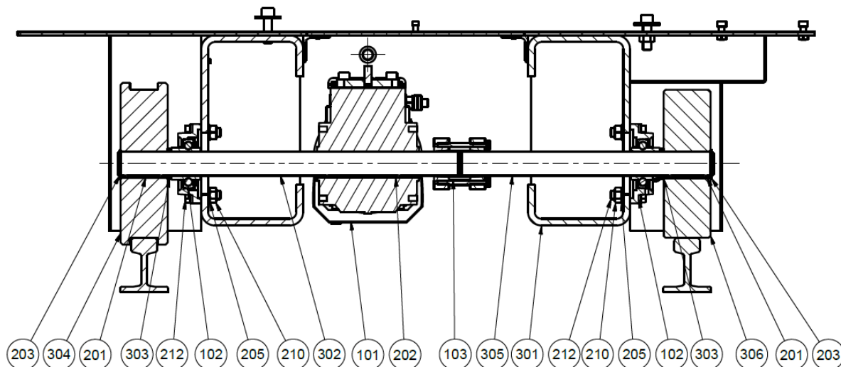
Slika 12. Pogon podvozja
