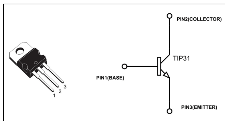
Slika 19: TIP 31C tranzistor [21]
