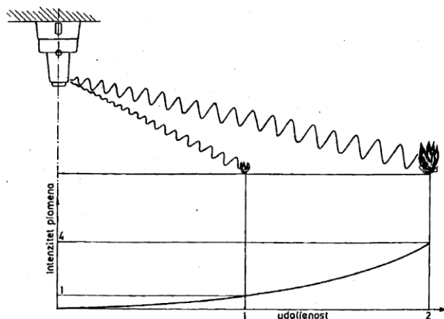
Slika 12. Prikaz udaljenosti javljača od plamena ovisno o intenzitetu plamena [1]
