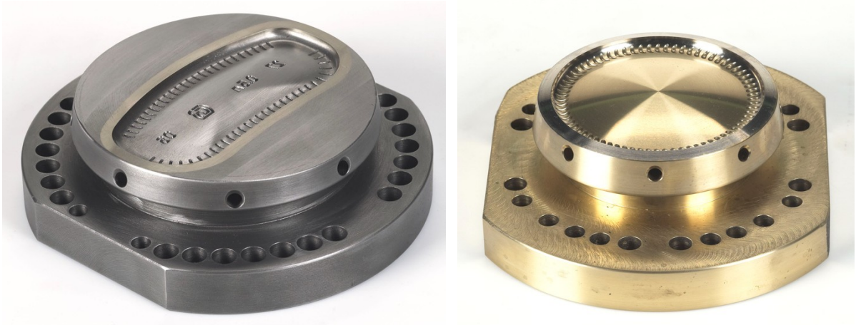
Slika 11. Dno kalupa [7]
