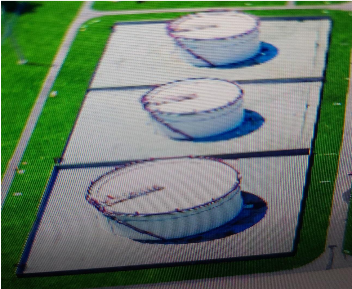
Slika 2. Spremnici sirove nafte s plivajućim krovom [3]
