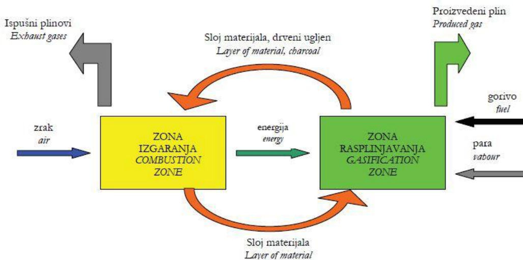
Slika 8. Osnovna shema postupka rasplinjavanja
