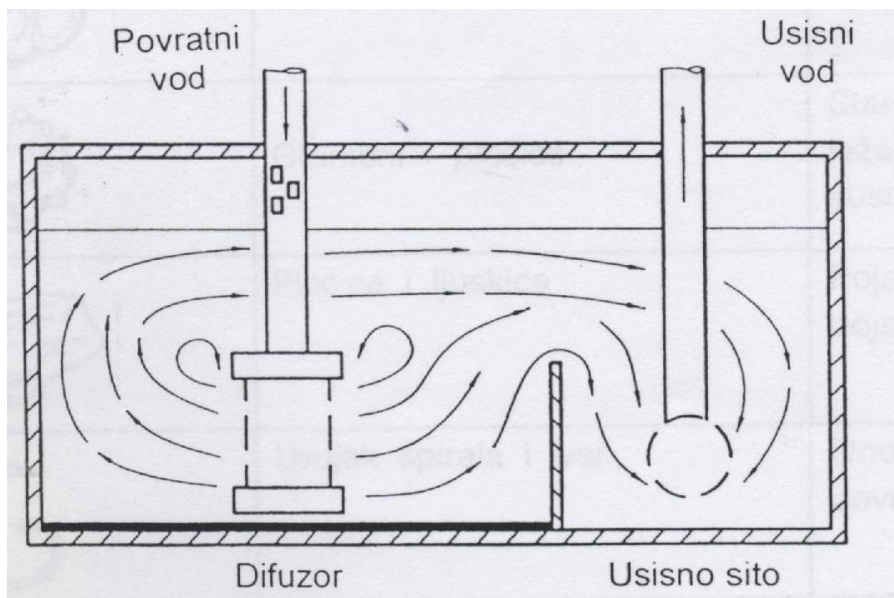
Slika 7. Unaprijedena konstrukcija spremnika ulja
