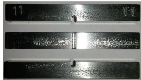
Slika 34 – Epruvete iz materijala Č4141
