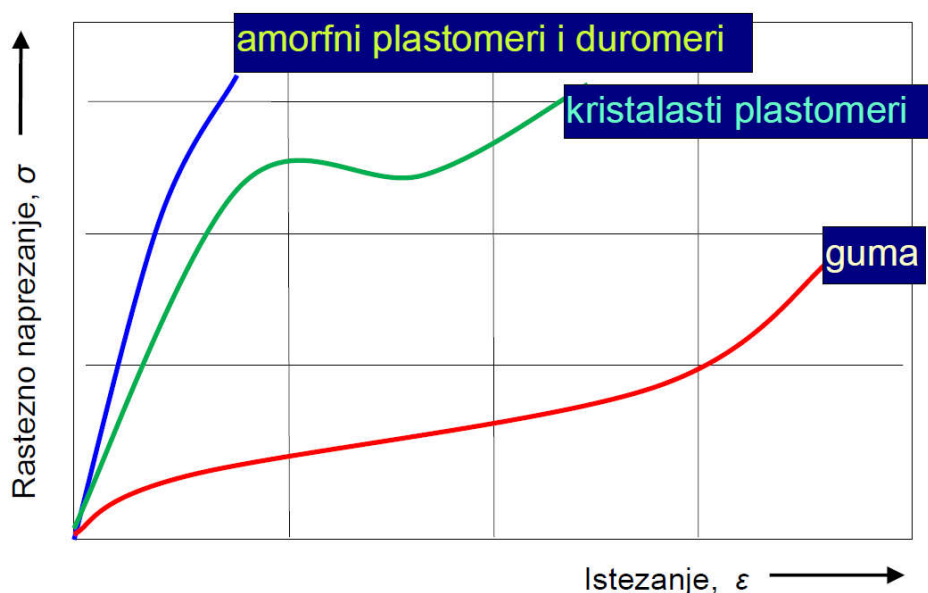
Slika 12. Karakteristični dijagram "naprezanje-istežanje" osnovnih skupina polimernih materijala[17]
