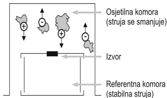
Slika 9. Ionizacijski detektor
