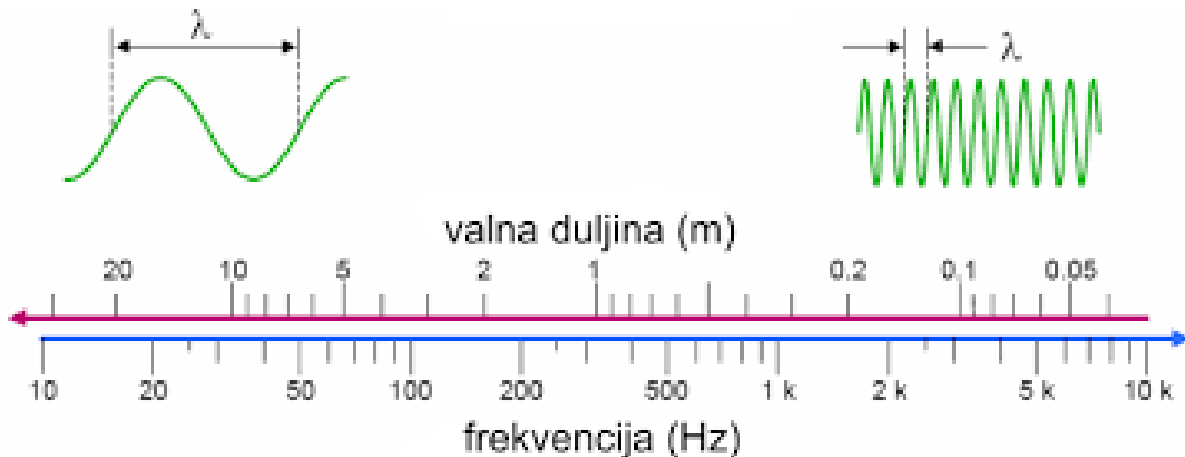
Slika 1. Graf zvuka
