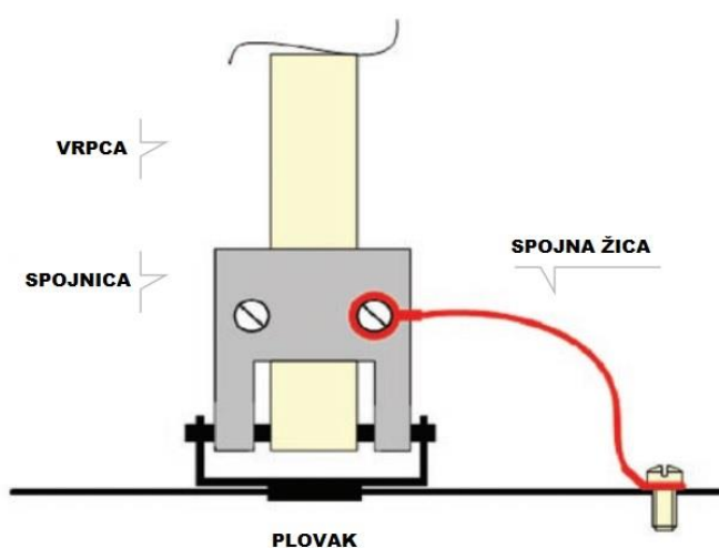
Slika 41: Preinaka koja je trebala biti poduzeta na plovku unutar spremnika s otapalom „ VM&P naphtha “ (ilustrativni primjer preporuke proizvođača plovaka koji su se koristili u kemijskom postrojenju „ Barton Solvents Inc. “) [19].
