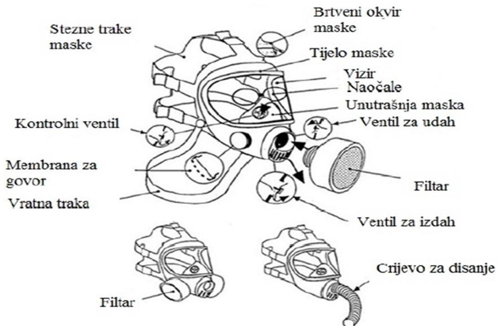
Sl. 3. Maska za cijelo lice sa dijelovima [4]
