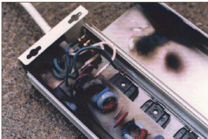
Sl.2. Kratki spoj unutar električne komponente [3]
