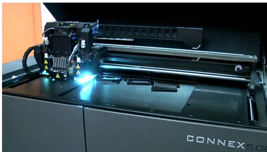
Slika 8. Polyjet pisač CONNEX 500 [8]
