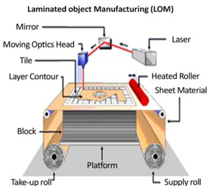
Slika 12. LOM postupak [12]
