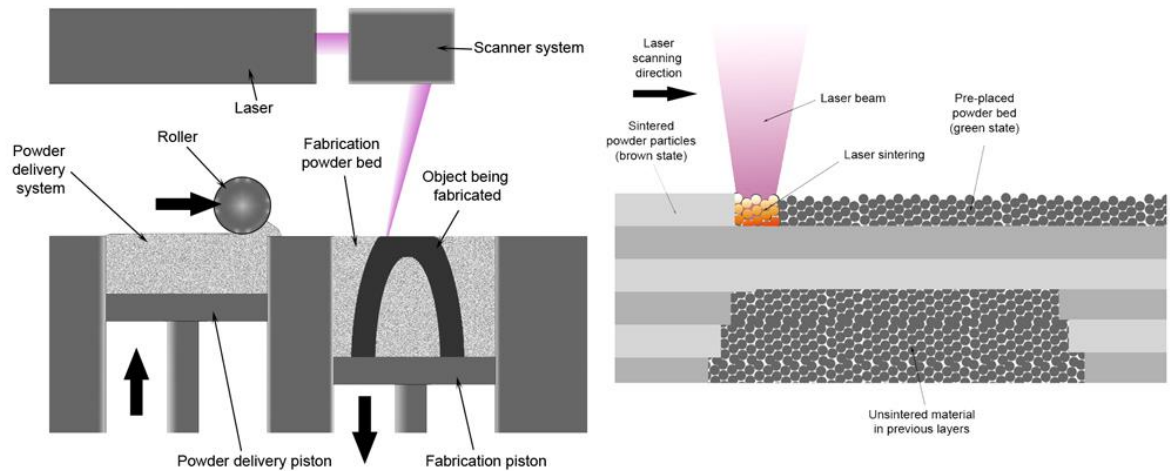
Slika 15. Princip rada SLS printera [15]
