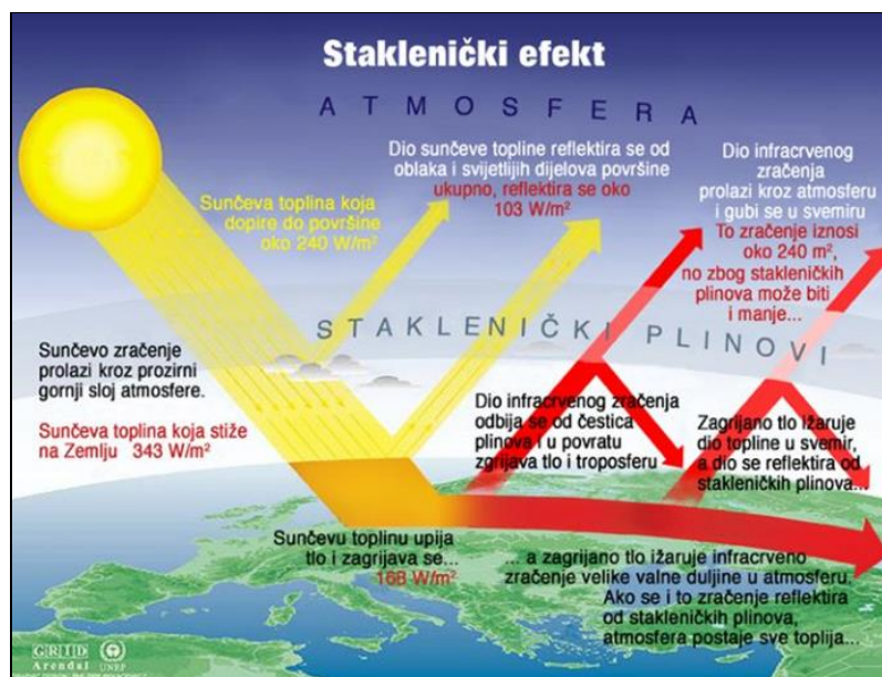
Slika 4: Staklenički efekt
