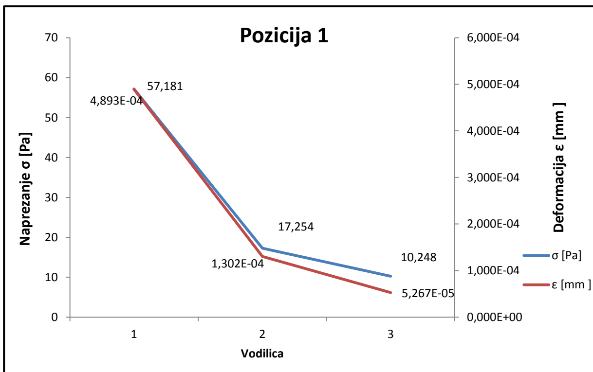
Slika 46. Grafički prikaz napreznja i deformacije (pozicija 1)
