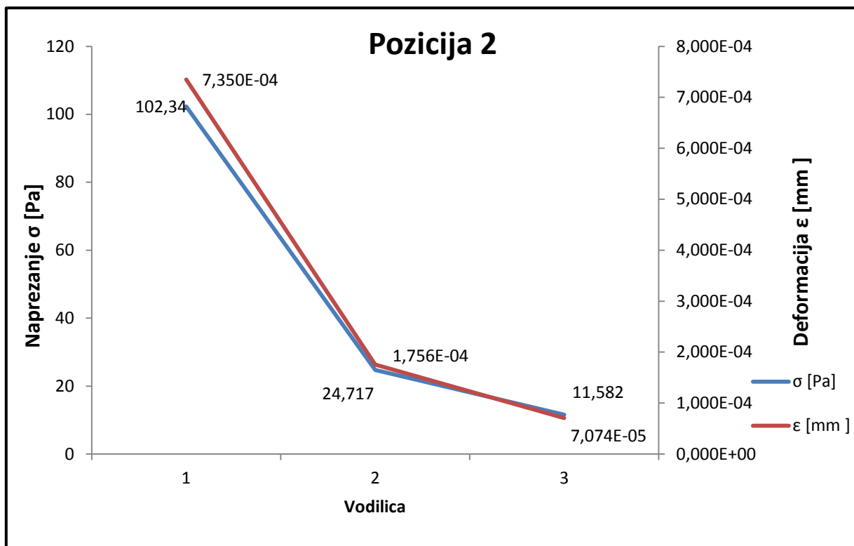
Slika 47. Grafički prikaz napreznja i deformacije (pozicija 2)
