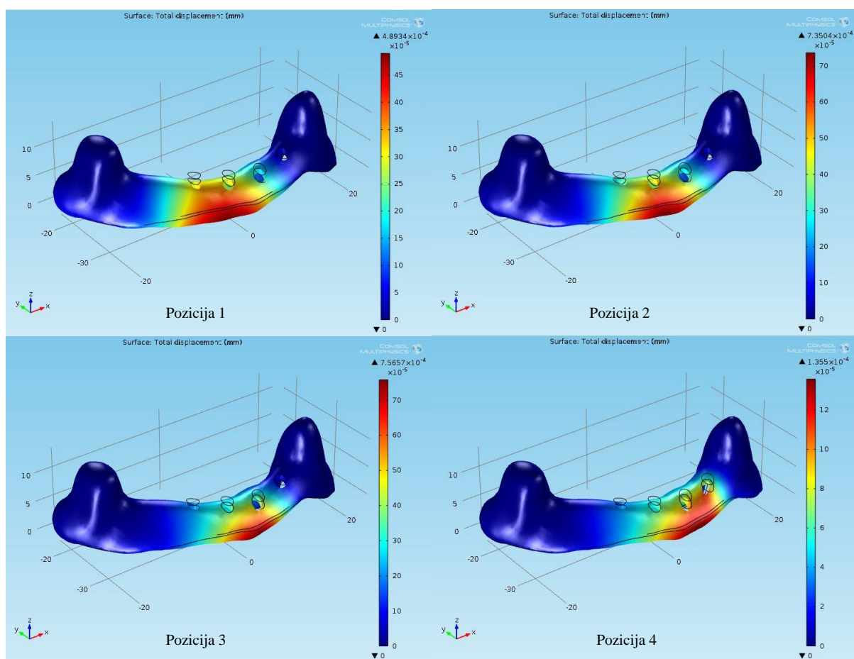
Slika 41. Prikaz deformacija vodilice debljine 1 mm (COMSOL)
