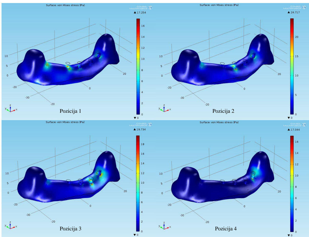
Slika 42. Prikaz naprežanja vodilice debljine 2 mm (COMSOL)
