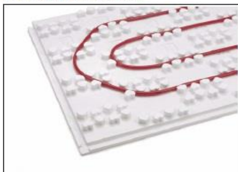
Sustav stiropomih ploča REHAU vario
