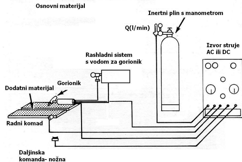
Slika 3. Shematski prikaz procesa i uređaja za TIG zavarivanje [10]
