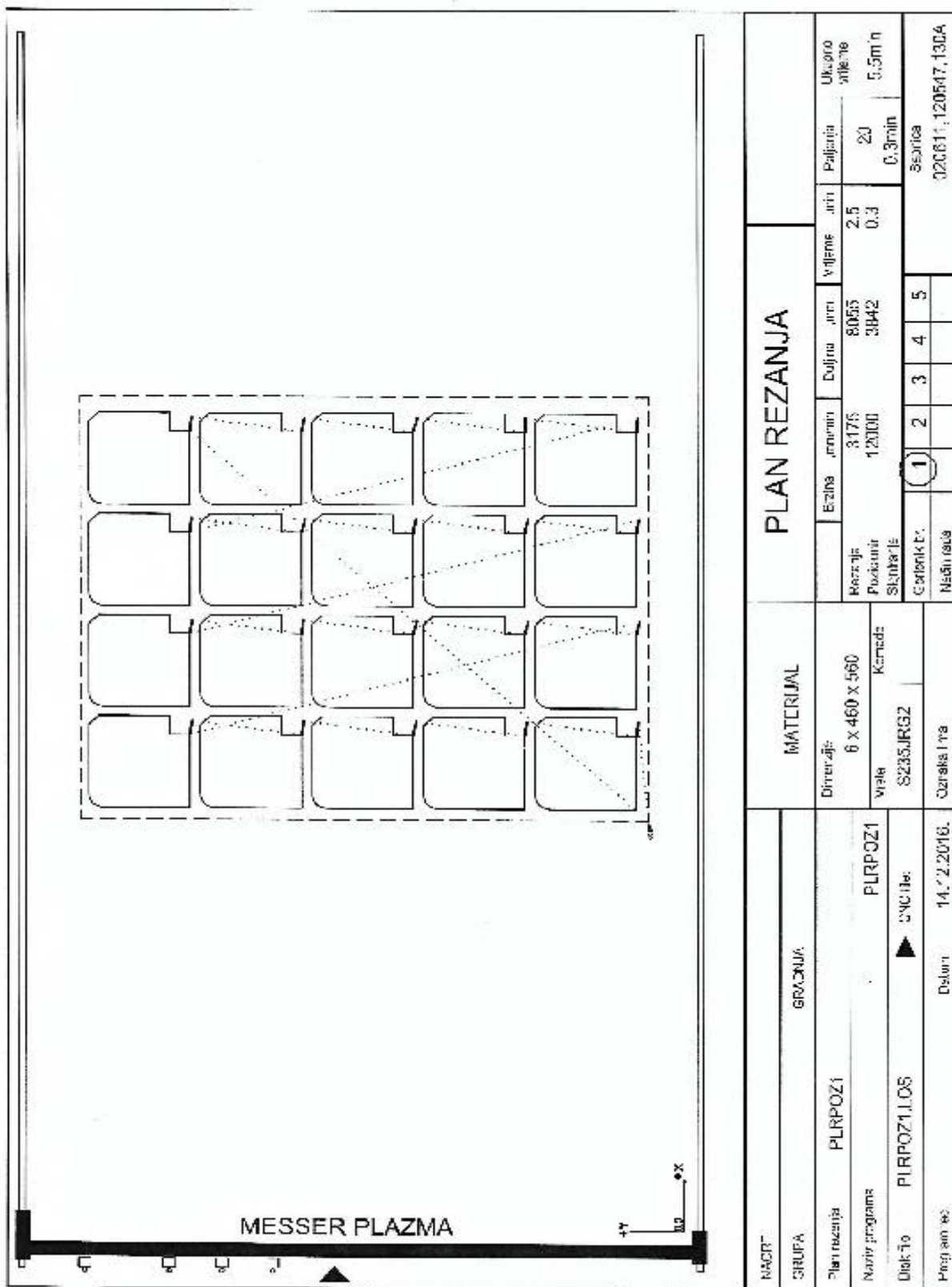
Sl. 37. Plan rezanja – izardak br.1. – REBRO
