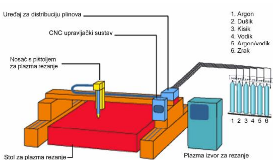
sl.9. Shema sustava za rezanje plazmom
