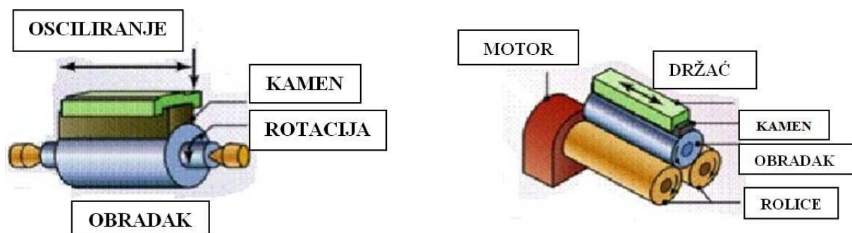
Slika 27. Postupak obrade superfinašem [27]
