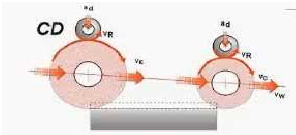
Slika 11. Neprekinuta obrada rezne površine brusa [11]
