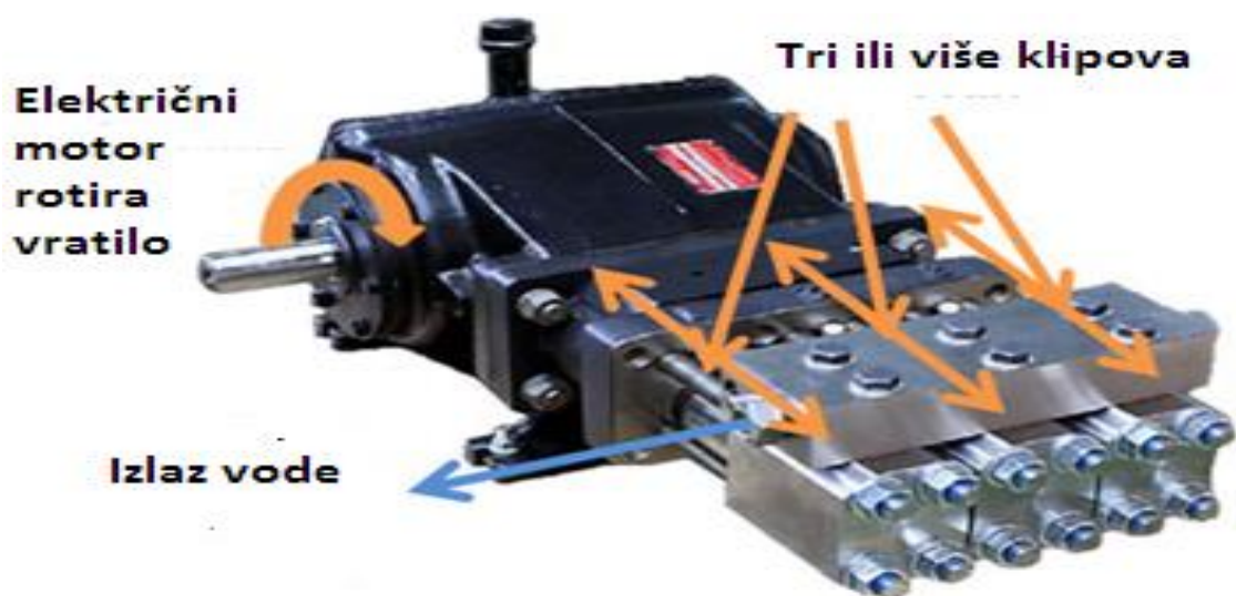
Slika 8. Klipna pumpa
