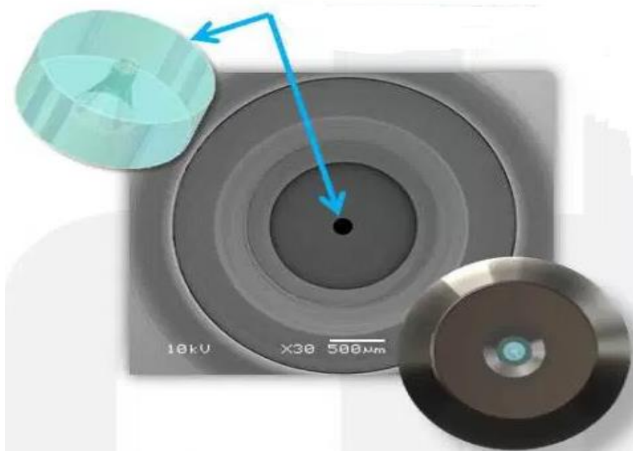
Slika 14. Dijamantna vodena mlaznica
