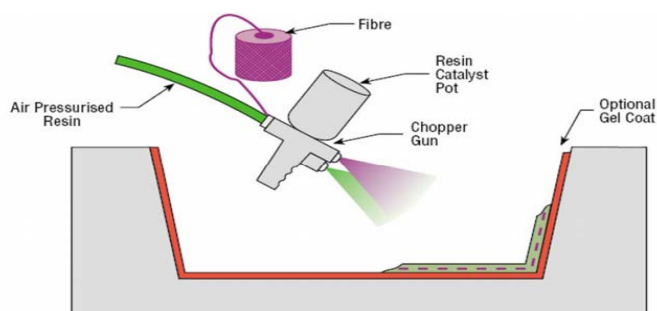
Slika 22.: Prikaz postupka oblikovanja naštrcavanjem [9]
