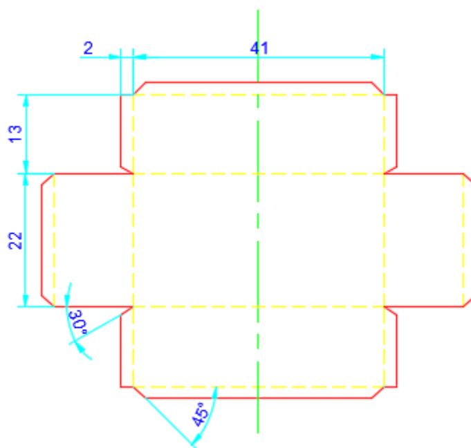
Slika 7. Skica kutije.
