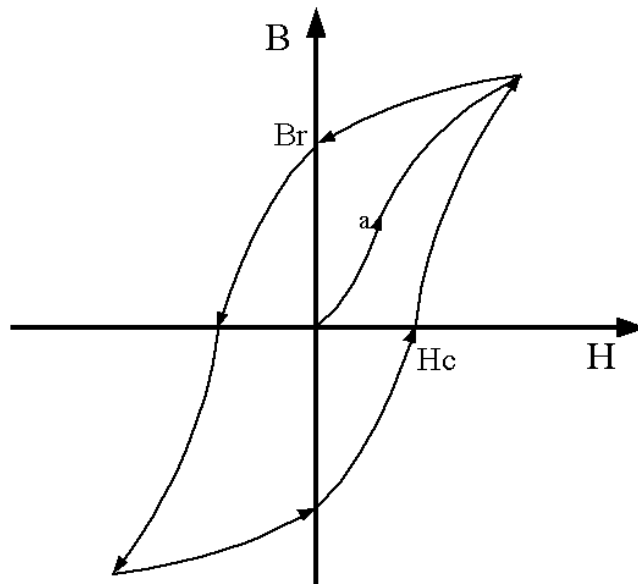
Slika. 20. Krivulja histereze
