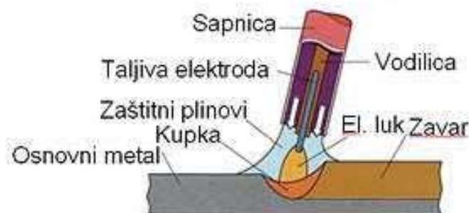
Slika 24. MIG/MAG zavarivanje
