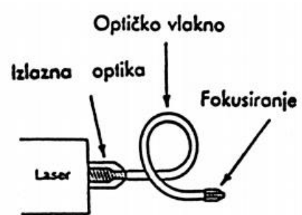
Slika 33. Optičko vođenje laserske zrake
