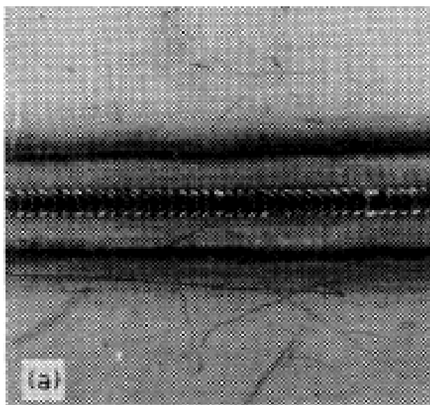
Slika 13. Preklapanje zavarenih spojeva kod pulsirajućeg TIG zavarivanja [7]
