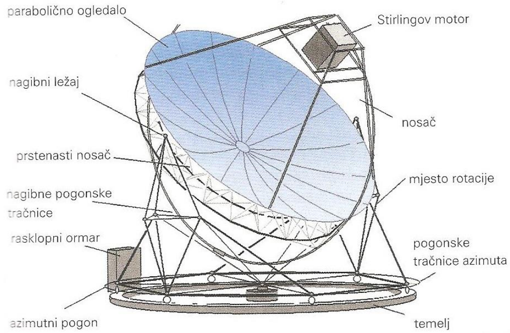
Slika 8.1. Sastavni dijelovi paraboličnog Stirlingova sustava [1]
