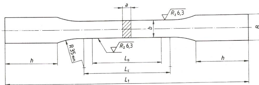
Slika 22 Dimenzije ispitnog uzorka za statički vlačni pokus.
