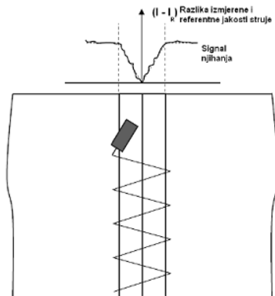
Slika 19. Shematski prikaz procesa zavarivanja kod kojeg nema devijacije žlijeba [28]
